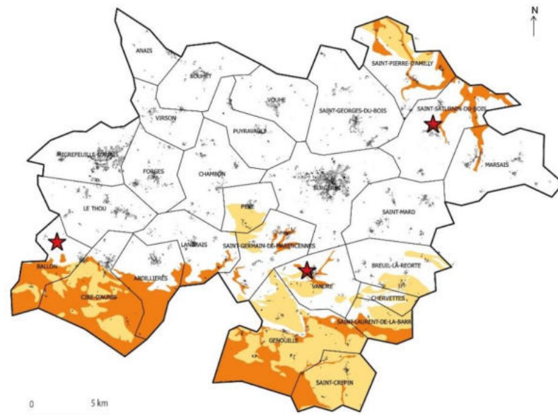
Aléas liés au retrait-gonflement des argiles
