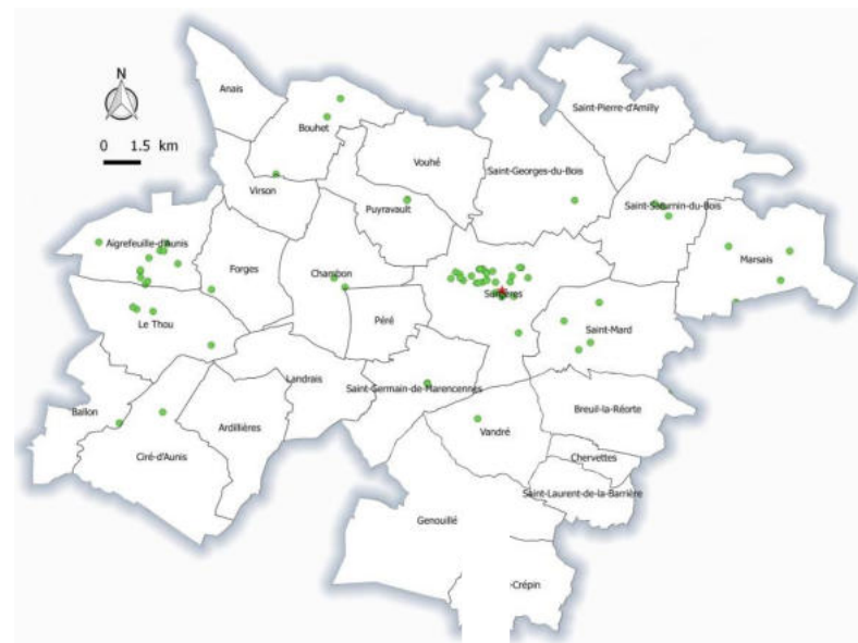
Sites BASOL et BASIAS sur Aunis Sud
