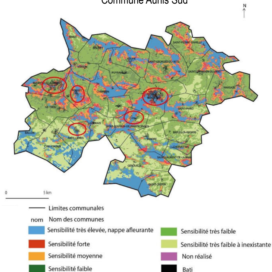
Aléa remontée de nappes dans la Communauté de Commune Aunis Sud
